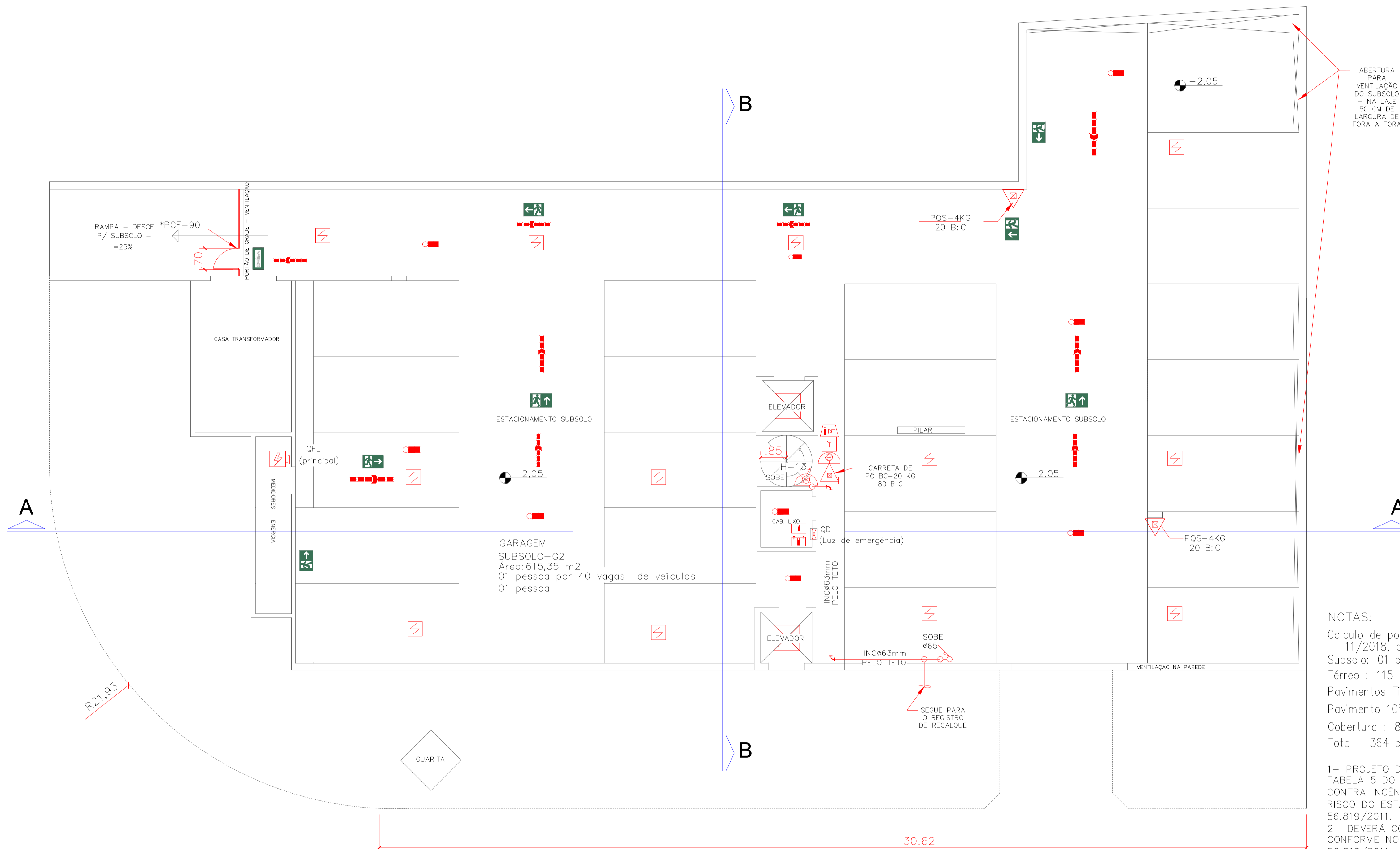
PLANTA BAIXA SUBSOLO ESCALA 1:75
